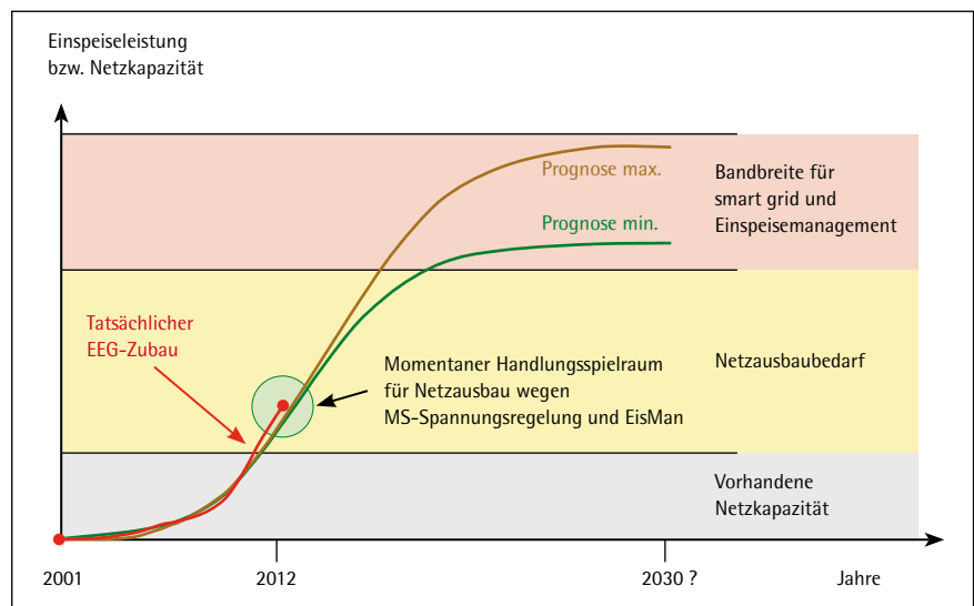
Bild 1: EEG-Zuwachs und Netzkapazität. Qualitative Darstellung
