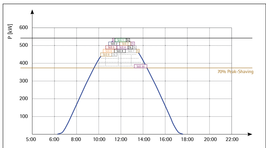
Bild 4: PV-Spitzenkappung alternativ durch smart local generation, Verbrauchersteuerung oder durch Elektrospeicher
