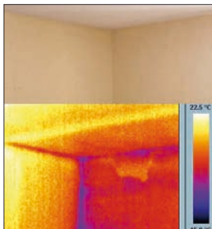
Bild 2: Wärmeverluste in der Zimmerecke
